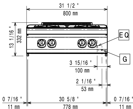
Przód
